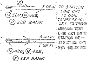
FIG. 2 BANK MULTIPLE NO. 711A, 701B, 711A, 711B OR 710E
