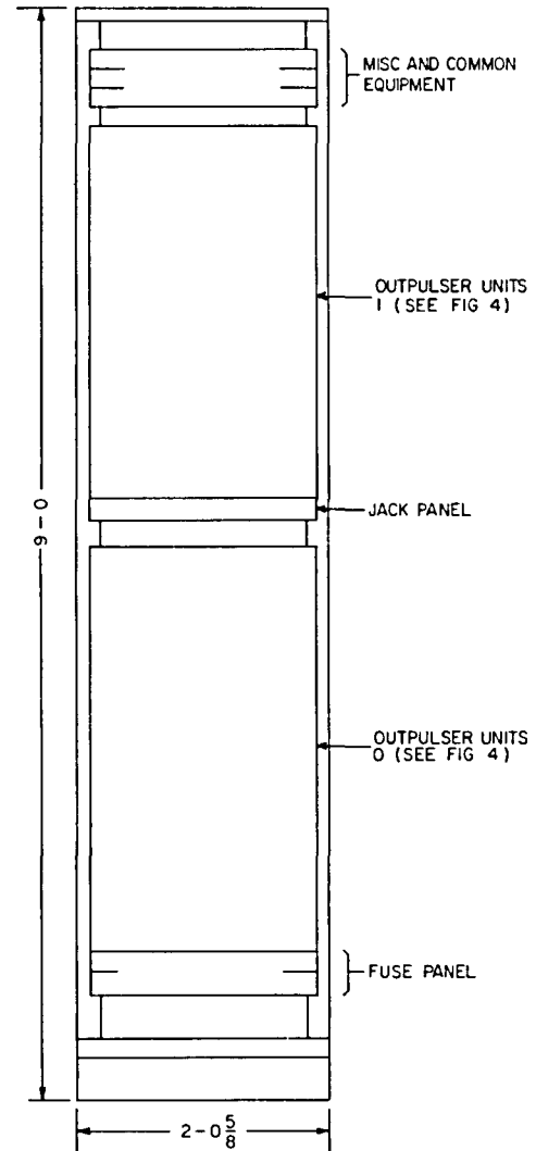
Fig 3—9-Foot Outputpulser Frame
