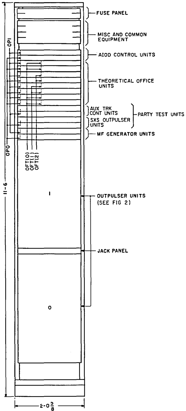
Fig 1—11-Foot 6-Inch Outpulser Frame
